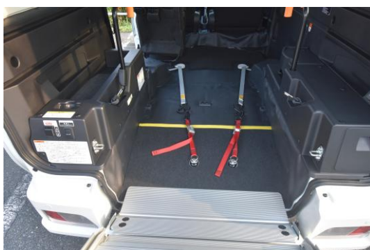
電動ウインチ、3点式シートベルト搭載
