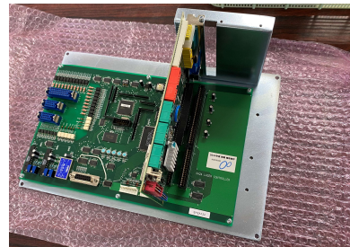
コントロールボード (64bit 対応) 最新のパソコンに対応し、画像データ 等処理能力が格段に上がった
