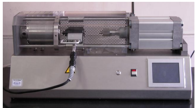
試験片作成用射出成形機
