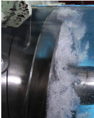
図1 ポンプに生じるキャビテーション
