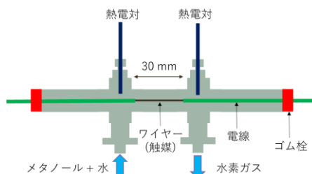
反応装置の概略図
