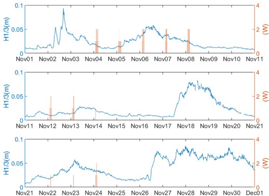
図3 岸壁における有義波高および発電量
