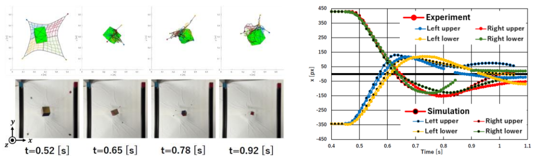
図6：自由落下するデブリの捕獲実験との比較結果
