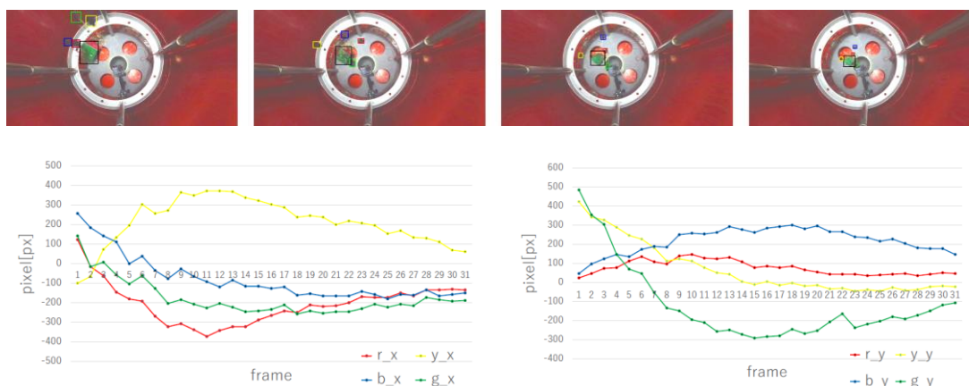
図8：自由落下するデブリの捕獲実験との比較結果
