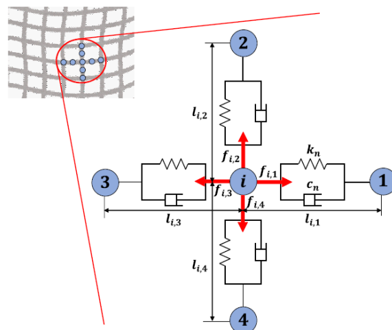
図1：ネット変形の動力学モデル
