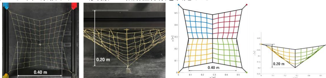
図5：ネット軸剛性係数の比較結果
