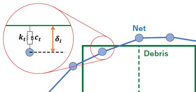
図2：ネットとデブリの接触力モデル
