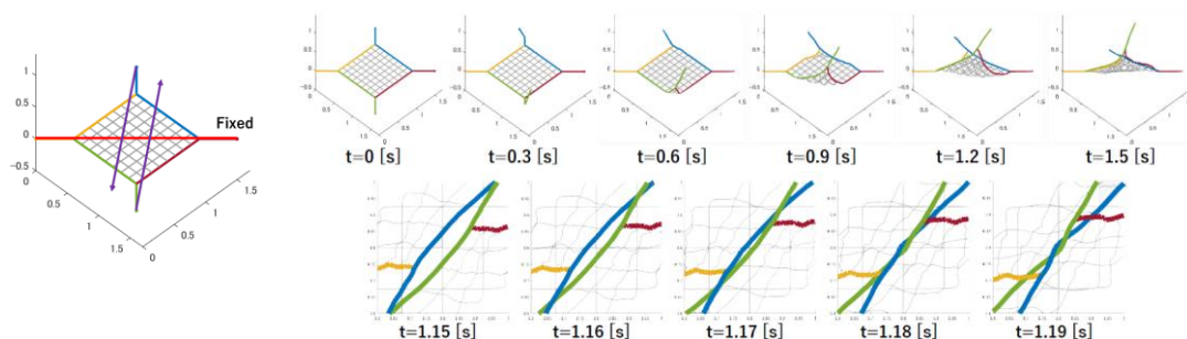
図4：ネット折り畳み動作のシミュレーション解析の結果
