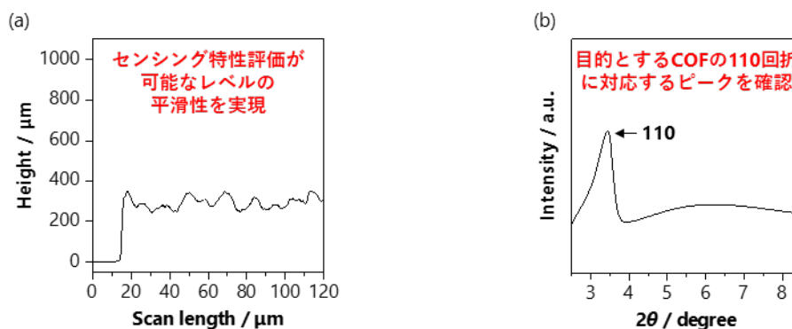
図1. 本研究で得られたCOF薄膜の構造解析例。(a) 触針式段差計による表面粗さの評価結果。平均膜厚が約300 nmであるに対し表面の凹凸は±50 nm程度であり、センシング特性評価が可能なレベルの平滑性をもつことが確認された。(b) X線回折測定による結晶性の評価結果。明確な回折ピークが想定した位置に観測され、成膜対象としたCOFの形成が確認された。
