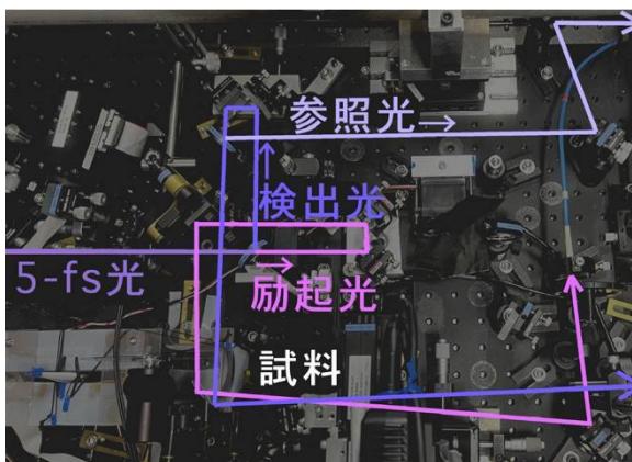
図1. 構築した検出光学系
