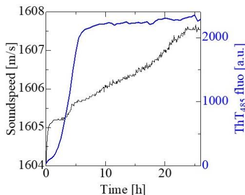
図 3. 超音波音速の変化と蛍光強度の同時計測結果
