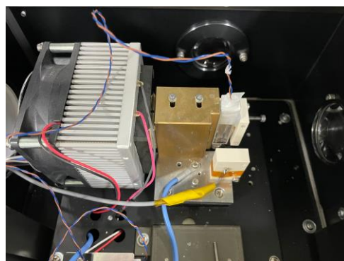
図 1. 構築した実験系
