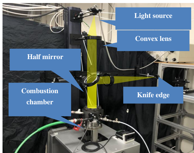
実験装置
