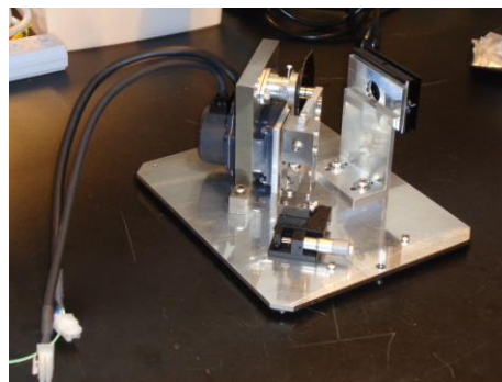
内部に取り付けた自作の摩擦試験機
