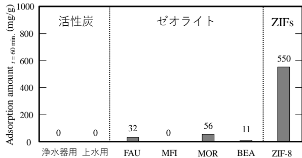
Fig. 2 各吸着剤の鉛イオン吸着容量
